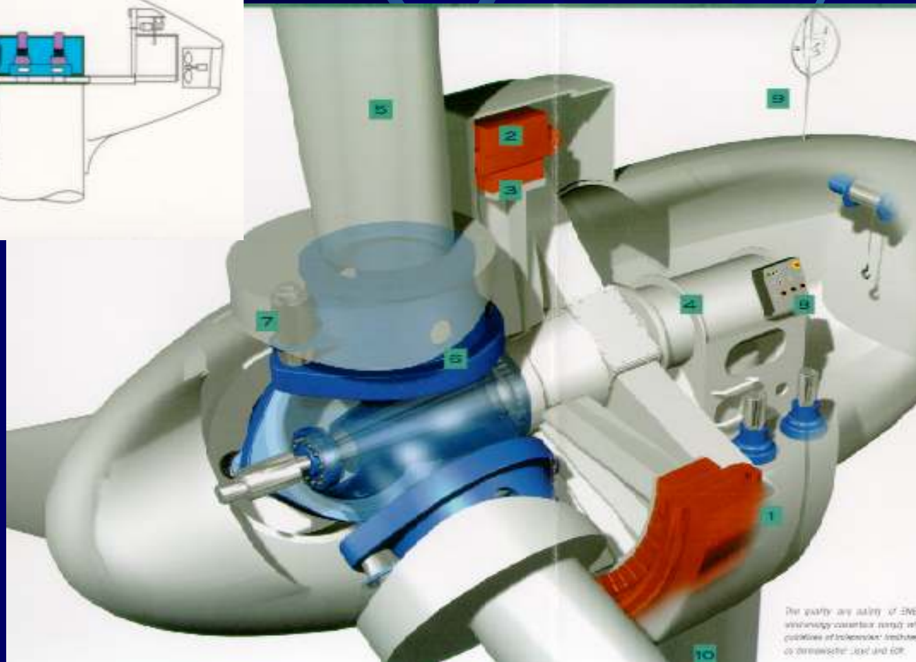
Przekrój gondoli siłowni firmy Enercon
